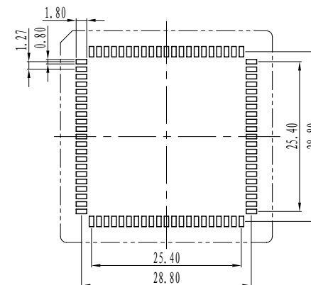
84PIN PCB LAYOUT
